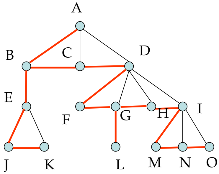
Arbre général
