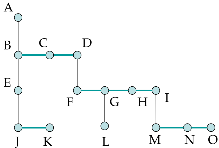
Arbre binaire
