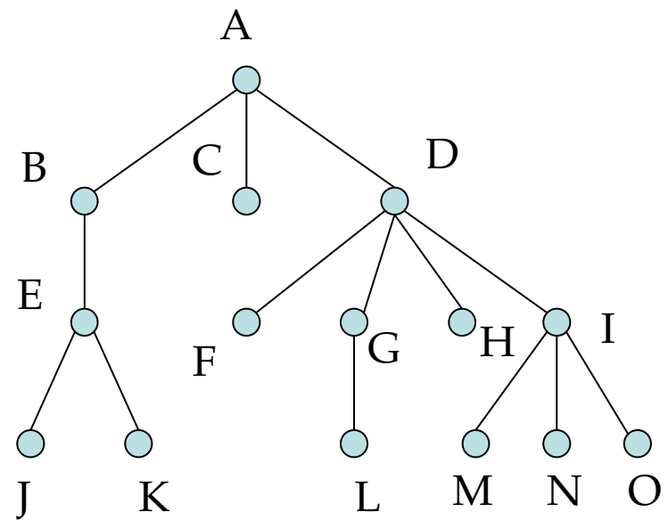
Arbre général
