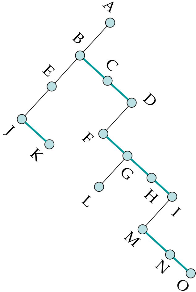
Arbre binaire
