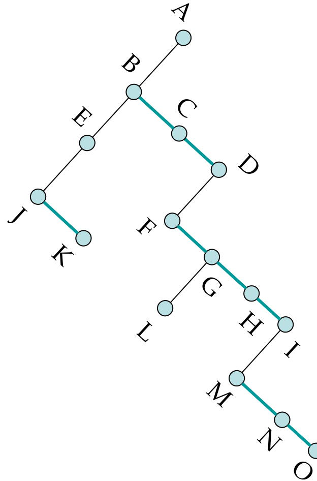
Arbre binaire
