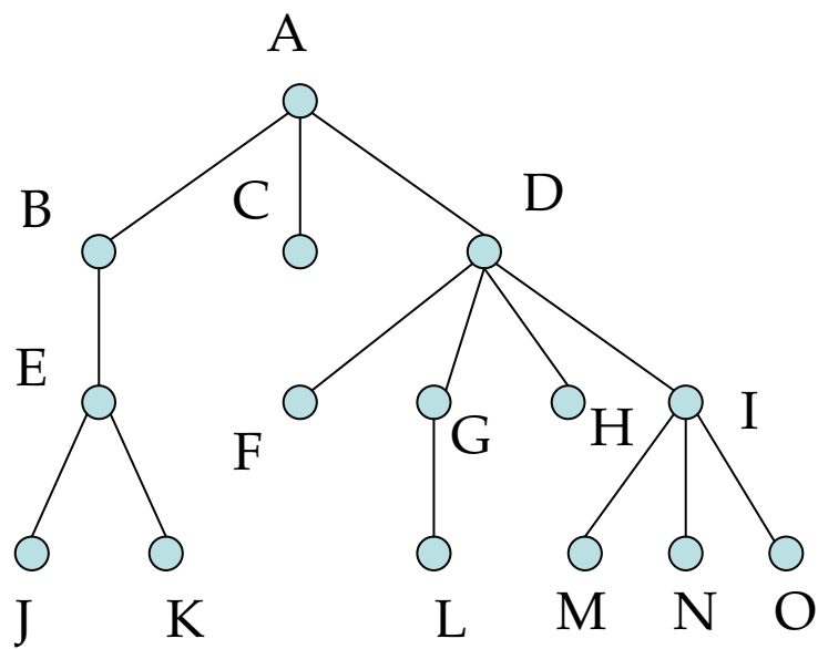
Arbre général
