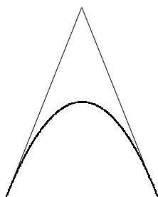
FIGURE 6: Courbe de Bézier : exemple
