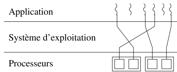
FIGURE 1.9 – Ordonnancement opportuniste dans un système d'exploitation.
