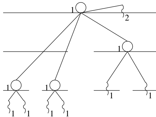
FIGURE 4.3 – Distribution de bulles et threads avec priorités.
