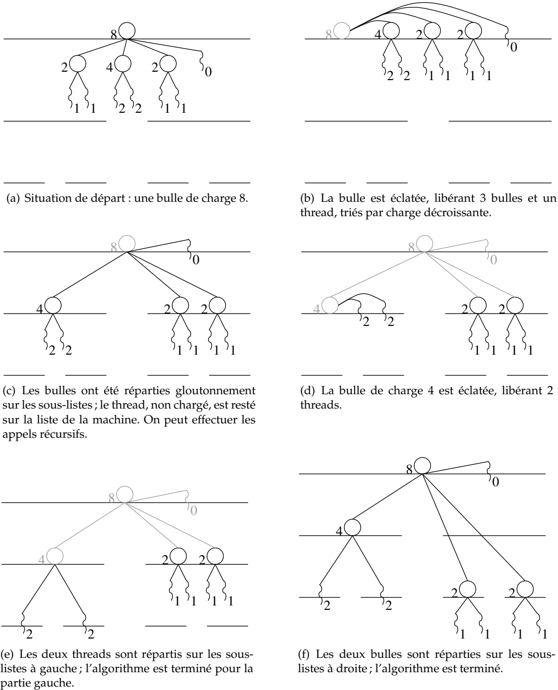
FIGURE 3.10 – Déroulement de l'ordonnancement Spread .
