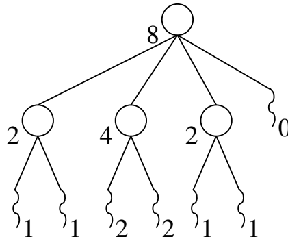
FIGURE 2.2 – Synthèse de l'estimation d'utilisation du temps processeur.
