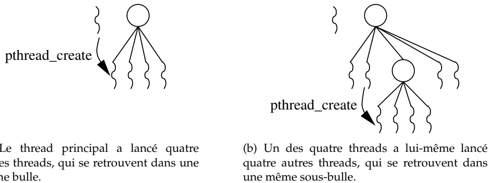
FIGURE 5.2 – Construction automatique de bulles à partir des relations de filiation POSIX.
