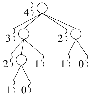
(c) Hiérarchie de bulles créée par un appel à fibonacci(4) .
