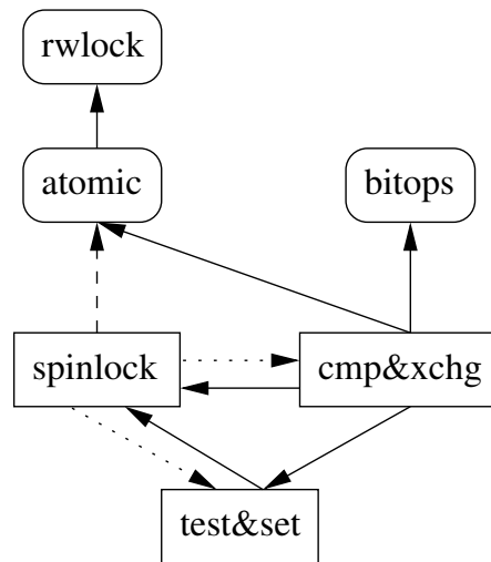
FIGURE 4.6 – Implémentations des opérations atomiques et verrous rotatifs.
