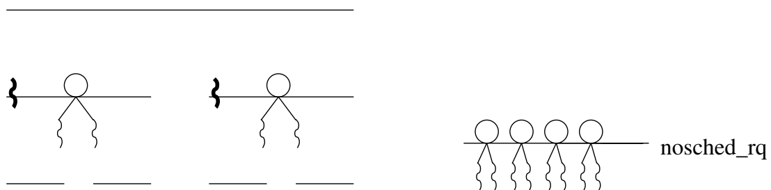
FIGURE 3.8 – Exécution de deux gang schedulers en parallèle (en gras), chacun piochant dans une liste commune une bulle à faire exécuter sur la partie de machine dont il a la charge.
