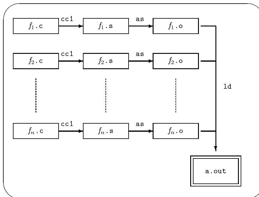
FIG. 4.1 – Schéma de la compilation d'un programme composé de plusieurs fichiers source.
