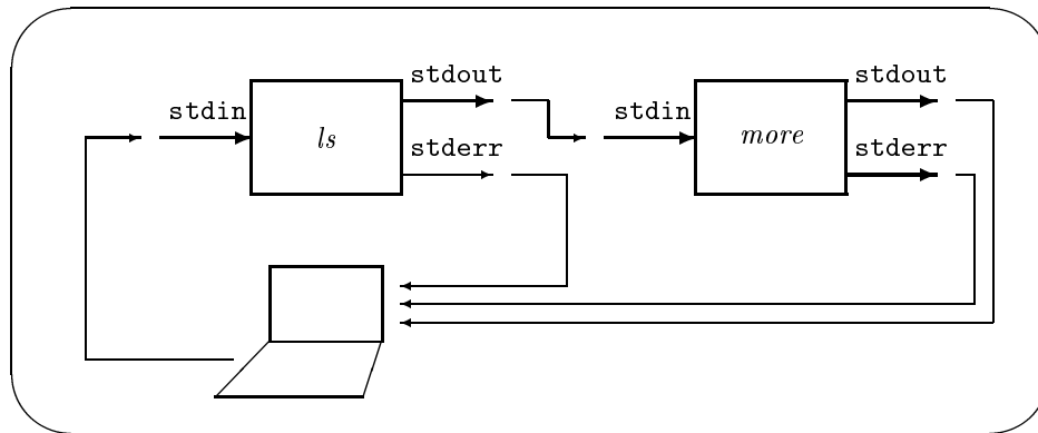
FIG. 2.3 – Résultat d'un pipe
